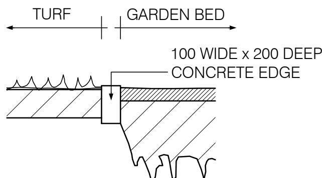
D GARDEN EDGE NTS
